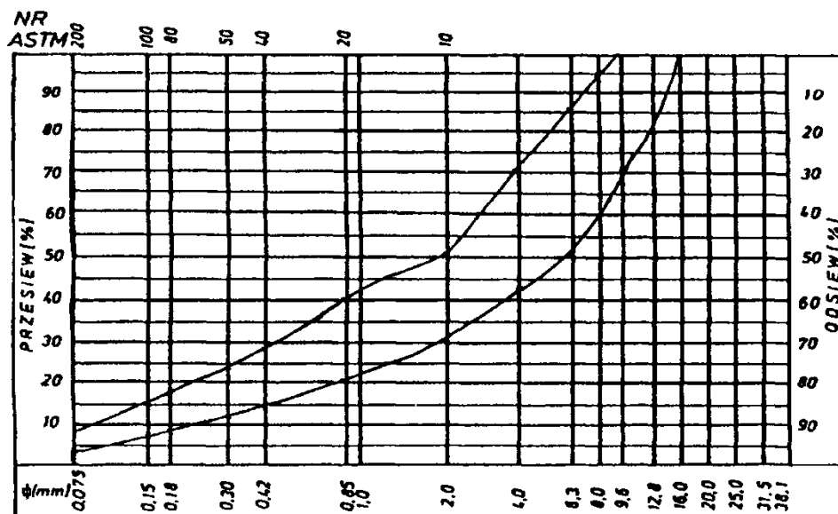
Rys. 2. Krzywe graniczne uziarnienia mieszanki mineralnej 0÷16 mm do warstwy wiążącej, wyrównawczej i wzmacniającej z betonu asfaltowego dla KR 1-2
