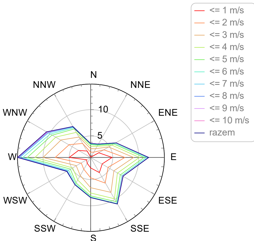
Rycina 4. Róża wiatrów roczna, stacja meteorologiczna w Kielcach
